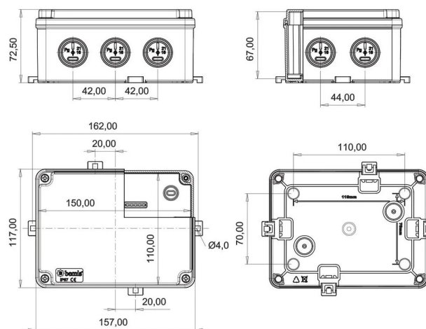
ГАБАРИТНЫЙ ЧЕРТЁЖ
