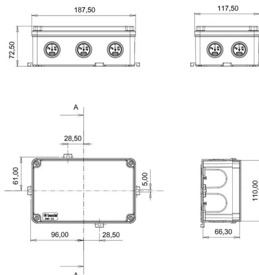
ГАБАРИТНЫЙ ЧЕРТЁЖ
