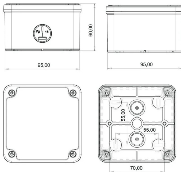
ГАБАРИТНЫЙ ЧЕРТЁЖ
