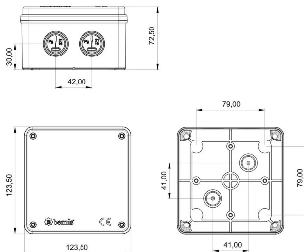
ГАБАРИТНЫЙ ЧЕРТЁЖ
