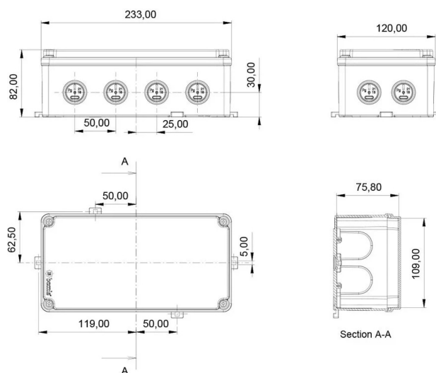
ГАБАРИТНЫЙ ЧЕРТЁЖ
