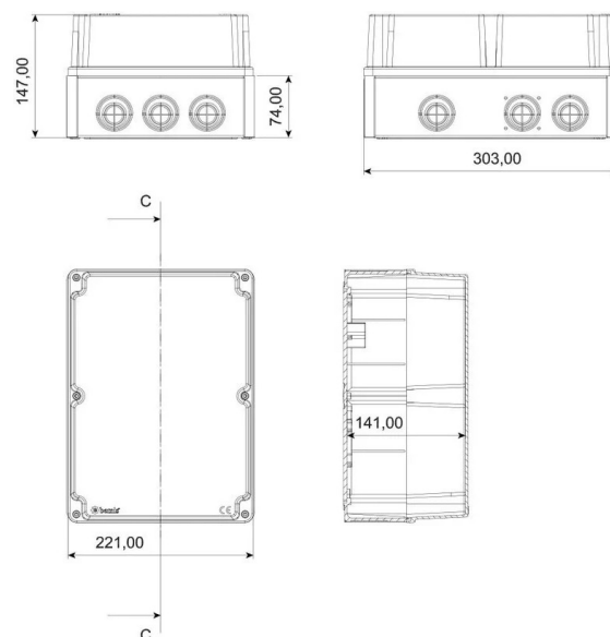
ГАБАРИТНЫЙ ЧЕРТЁЖ
