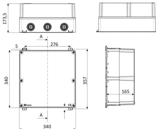
ГАБАРИТНЫЙ ЧЕРТЁЖ
