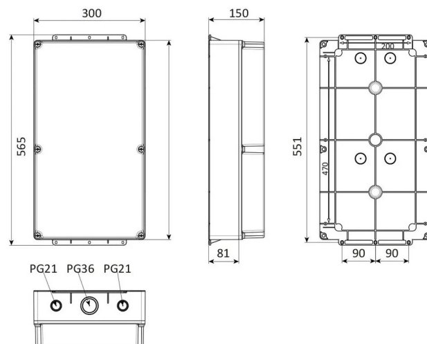
ГАБАРИТНЫЙ ЧЕРТЁЖ
