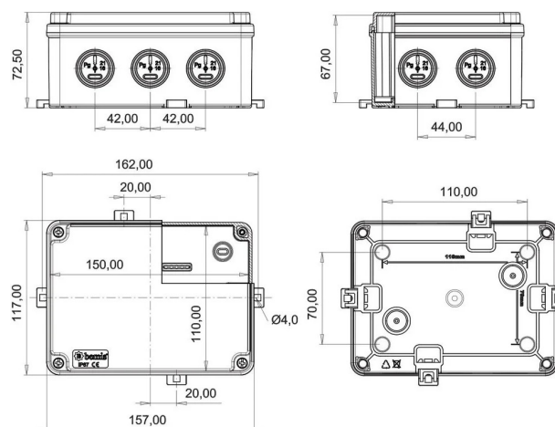
ГАБАРИТНЫЙ ЧЕРТЁЖ
