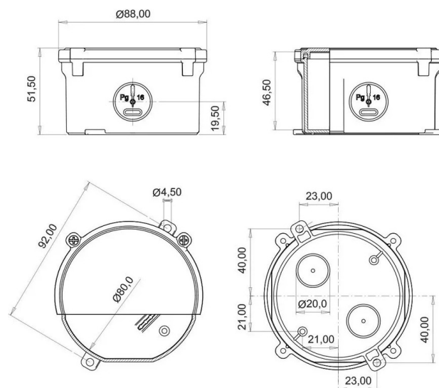
ГАБАРИТНЫЙ ЧЕРТЁЖ
