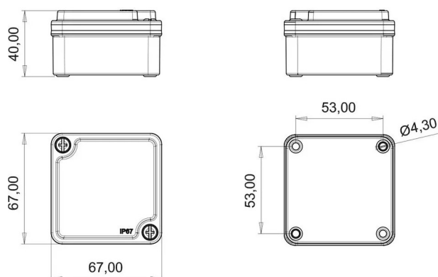
ГАБАРИТНЫЙ ЧЕРТЁЖ
