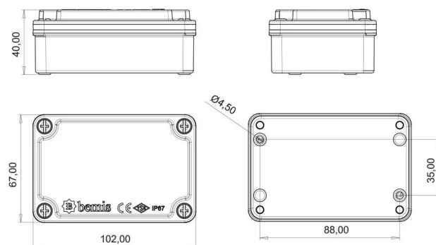
ГАБАРИТНЫЙ ЧЕРТЁЖ
