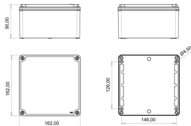
ГАБАРИТНЫЙ ЧЕРТЁЖ
