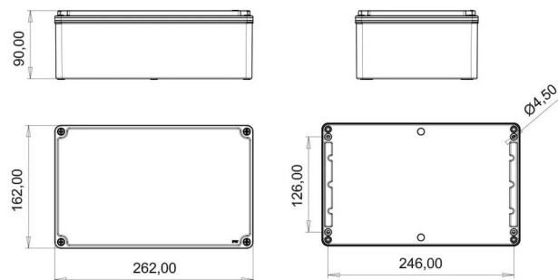
ГАБАРИТНЫЙ ЧЕРТЁЖ
