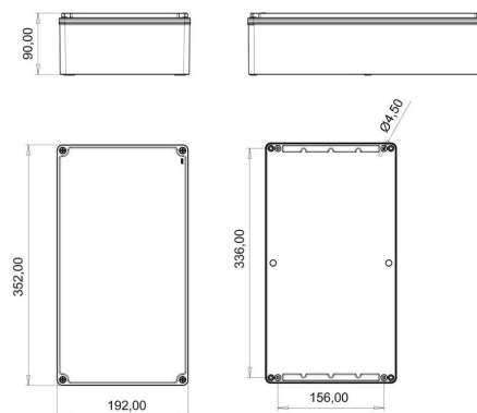
ГАБАРИТНЫЙ ЧЕРТЁЖ
