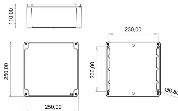
ГАБАРИТНЫЙ ЧЕРТЁЖ
