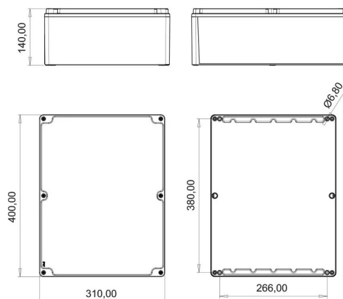
ГАБАРИТНЫЙ ЧЕРТЁЖ
