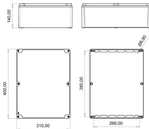
ГАБАРИТНЫЙ ЧЕРТЁЖ
