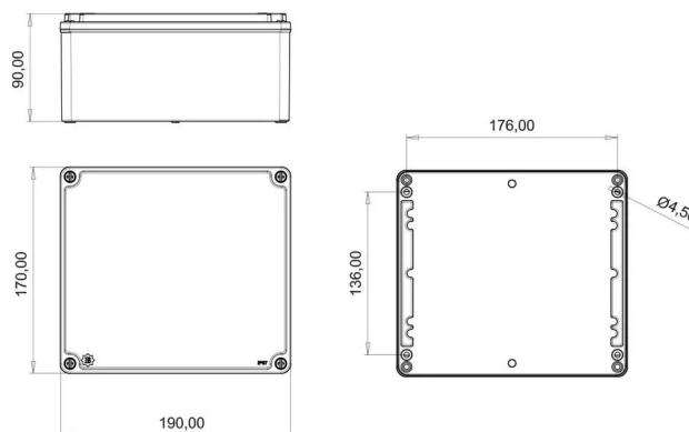
ГАБАРИТНЫЙ ЧЕРТЁЖ
