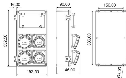
ГАБАРИТНЫЙ ЧЕРТЁЖ
