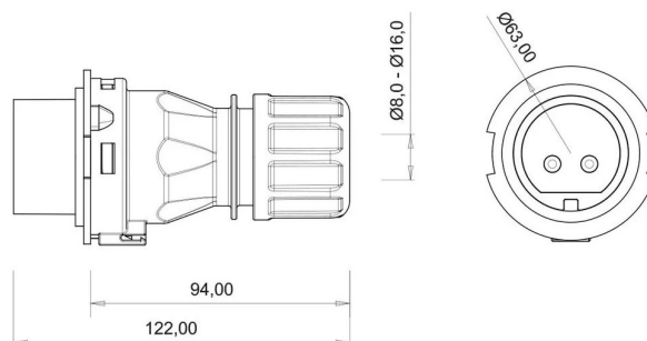
ГАБАРИТНЫЙ ЧЕРТЁЖ
