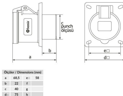
ГАБАРИТНЫЙ ЧЕРТЁЖ
