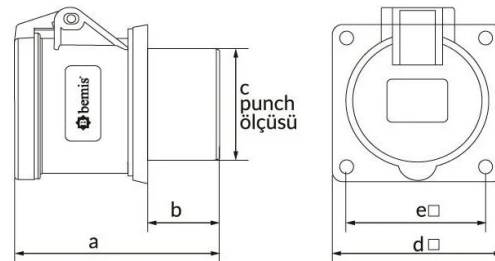
ГАБАРИТНЫЙ ЧЕРТЁЖ
