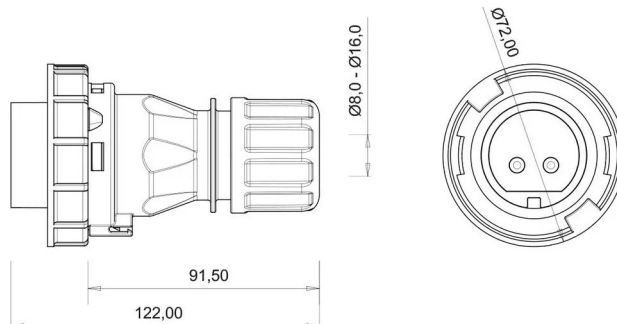
ГАБАРИТНЫЙ ЧЕРТЁЖ
