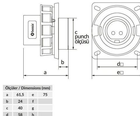
ГАБАРИТНЫЙ ЧЕРТЁЖ
