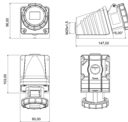
ГАБАРИТНЫЙ ЧЕРТЁЖ
