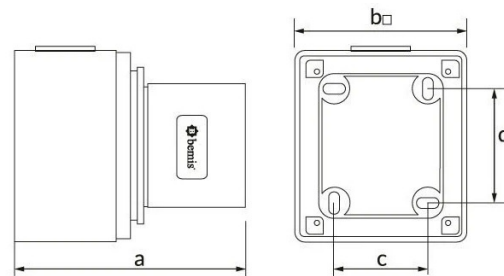
ГАБАРИТНЫЙ ЧЕРТЁЖ
