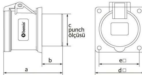
ГАБАРИТНЫЙ ЧЕРТЁЖ
