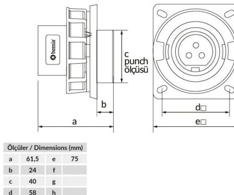
ГАБАРИТНЫЙ ЧЕРТЁЖ
