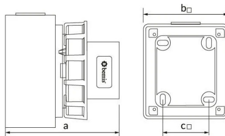
Ölçüler / Dimensions (mm)
