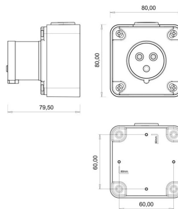
ГАБАРИТНЫЙ ЧЕРТЁЖ
