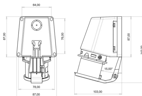
ГАБАРИТНЫЙ ЧЕРТЁЖ
