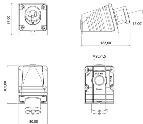
ГАБАРИТНЫЙ ЧЕРТЁЖ
