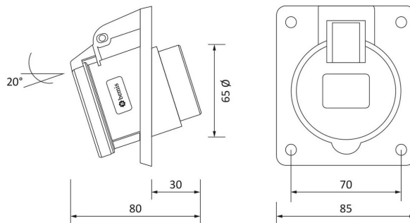
ГАБАРИТНЫЙ ЧЕРТЁЖ
