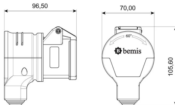
ГАБАРИТНЫЙ ЧЕРТЁЖ
