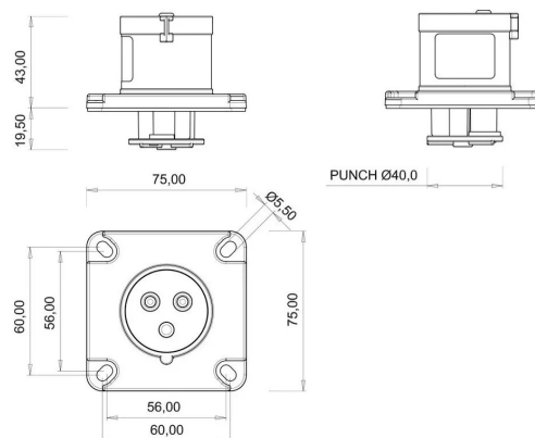
ГАБАРИТНЫЙ ЧЕРТЁЖ
