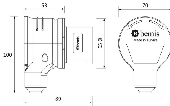
ГАБАРИТНЫЙ ЧЕРТЁЖ
