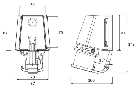
ГАБАРИТНЫЙ ЧЕРТЁЖ
