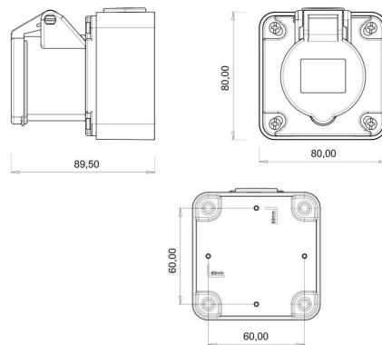
ГАБАРИТНЫЙ ЧЕРТЁЖ
