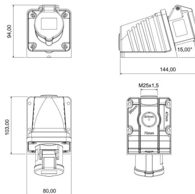
ГАБАРИТНЫЙ ЧЕРТЁЖ
