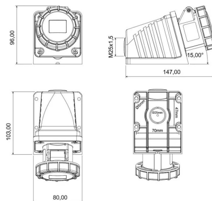
ГАБАРИТНЫЙ ЧЕРТЁЖ
