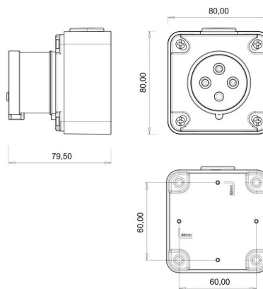
ГАБАРИТНЫЙ ЧЕРТЁЖ
