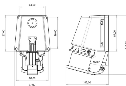
ГАБАРИТНЫЙ ЧЕРТЁЖ
