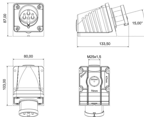
ГАБАРИТНЫЙ ЧЕРТЁЖ
