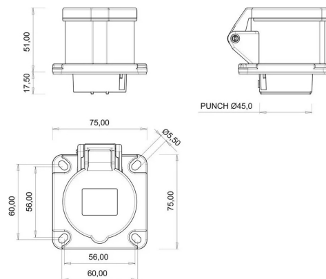
ГАБАРИТНЫЙ ЧЕРТЁЖ
