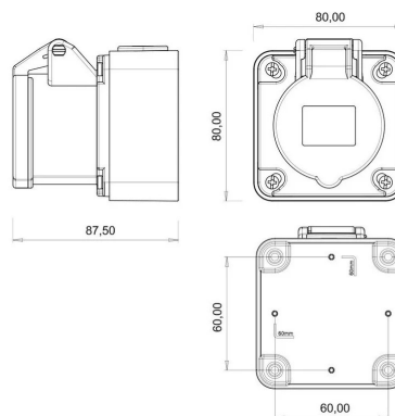
ГАБАРИТНЫЙ ЧЕРТЁЖ
