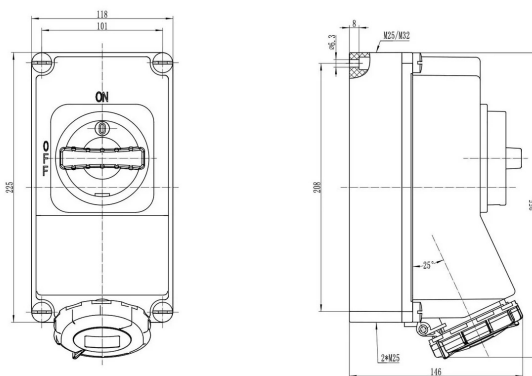
ГАБАРИТНЫЙ ЧЕРТЁЖ
