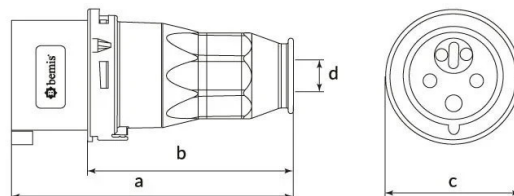
ГАБАРИТНЫЙ ЧЕРТЁЖ
