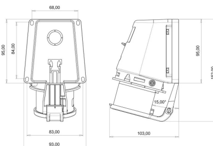
ГАБАРИТНЫЙ ЧЕРТЁЖ
