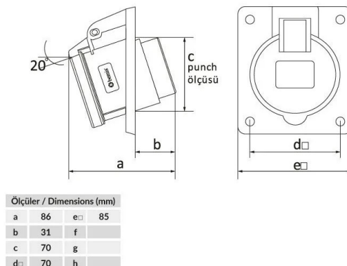
ГАБАРИТНЫЙ ЧЕРТЁЖ
